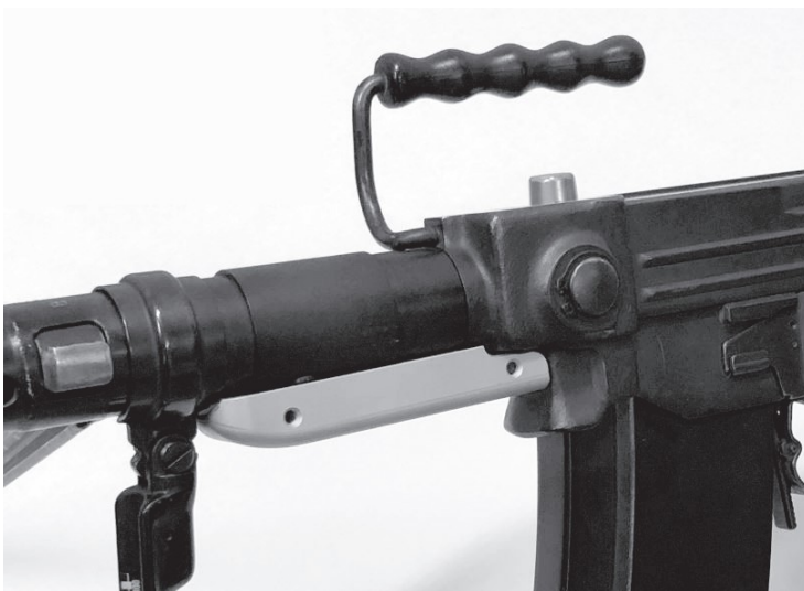
Bild 32: Handschutz zu Stgw 57
