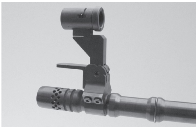
Bild 25: Kornträger als Visierverlängerung (Laufmontage), diverse Fabrikate
