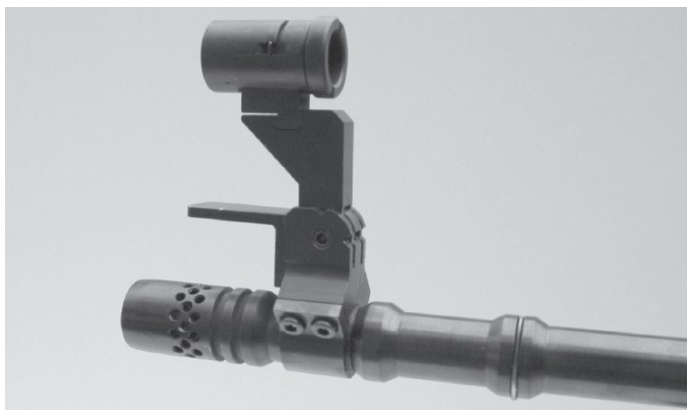
Figura 25: portamirino come prolungamento della linea di mira (montaggio sulla canna), diversi modelli
