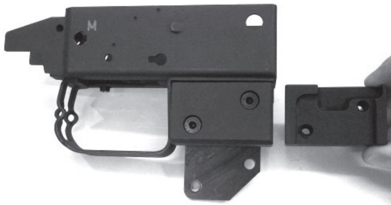
Bild 30: Griffadapter zu Stgw 57
