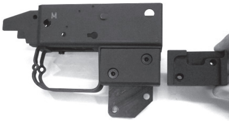
Figure 30: Adaptateur de poignée pour F ass 57
