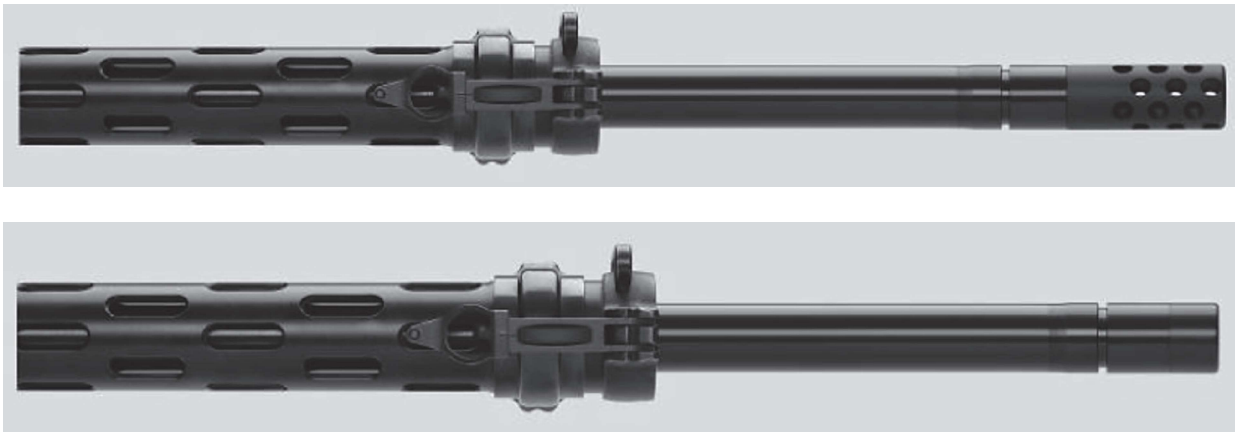
Bild 35: Sportlauf mit und ohne Feuerscheindämpfer zu Stgw 57
