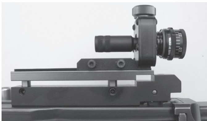
Figure 27: Porte dioptre pour F ass 57 pour le montage de dioptres à l'épreuve des vibrations de tir produits divers
