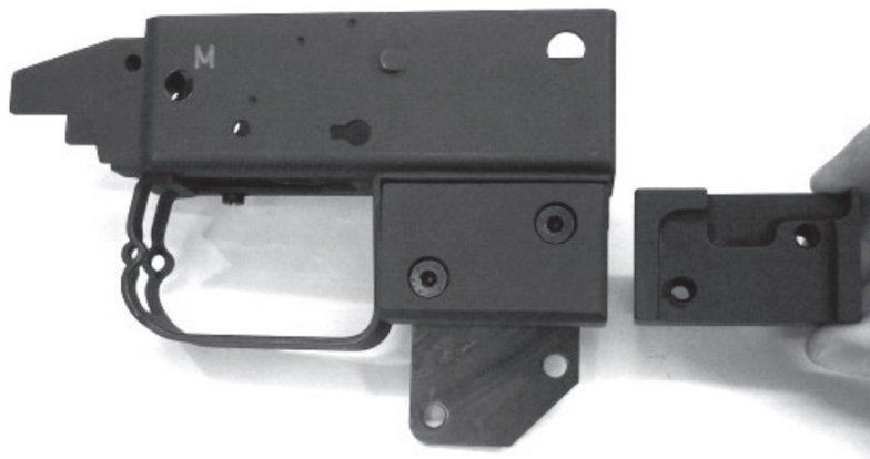
Figura 30: adattatore per l'impugnatura per F ass 57
